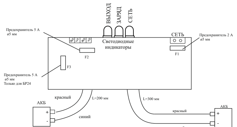
Рисунок 2 – Схема подключения платы бокса
